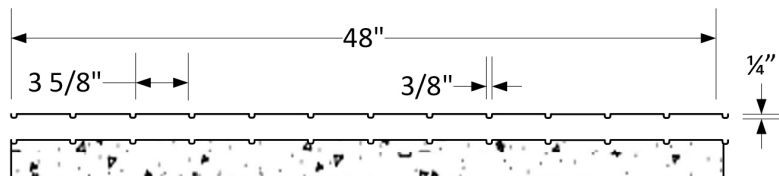
Section A-A
