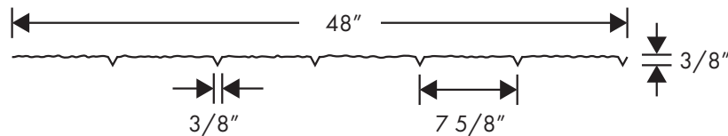
Section A-A
